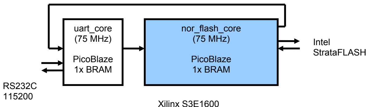
Obrázek 7: Blokové schéma funkčního vzorku s NOR_FLASH_CORE
