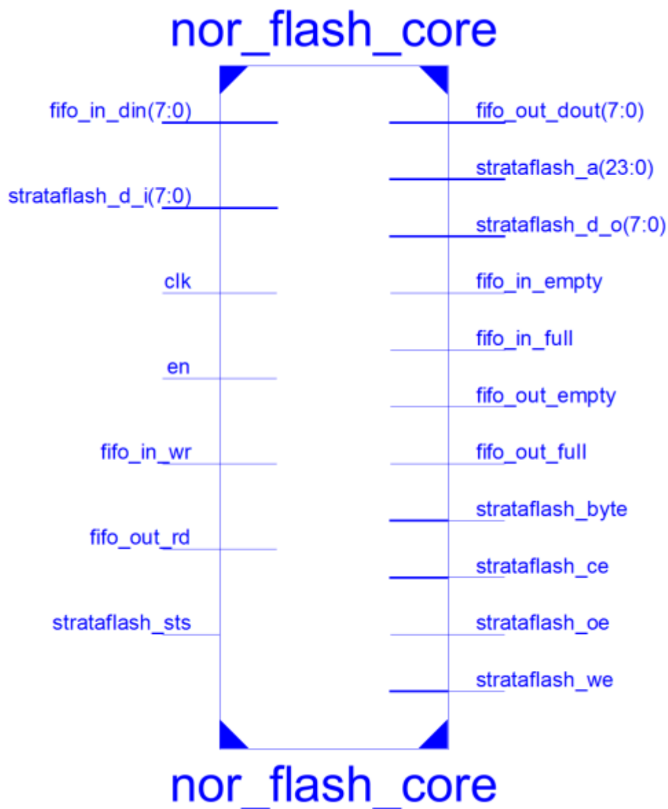
Obrázek 6 Modul nor_flash_core v ISE 13.2
