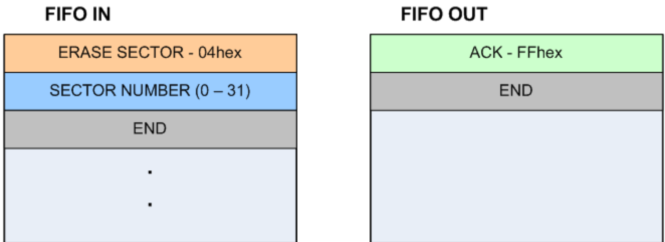
Obrázek 4 Sekvence příkazu ERASE SECTOR
