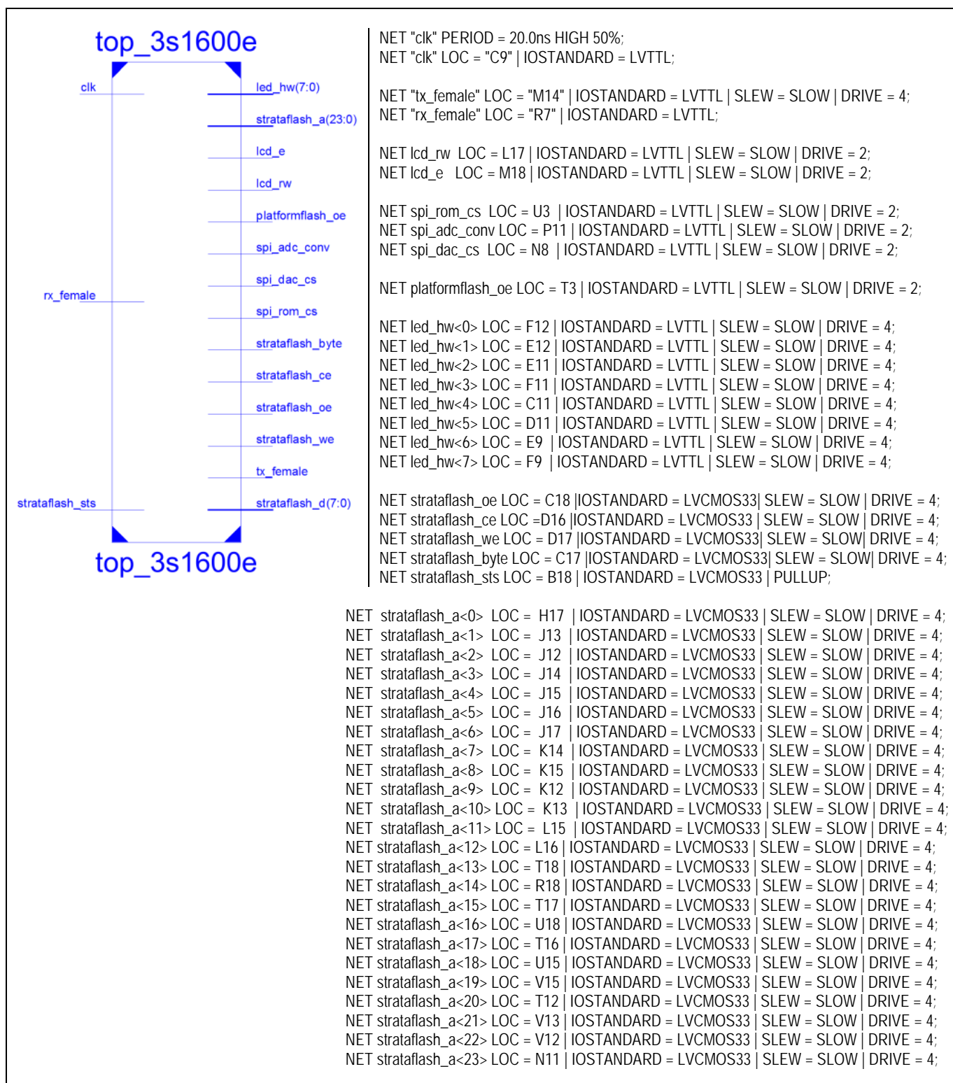
Tabulka 5 – Vstupy a výstupy demonstrátoru funkčního vzorku nor_flash_core na desce S3E1600
