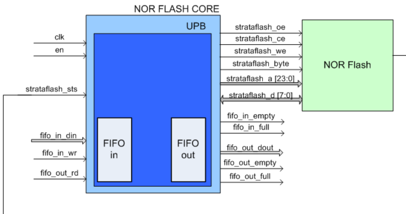
Obrázek 1 Blokové schéma modulu řadiče paměti NOR Flash
